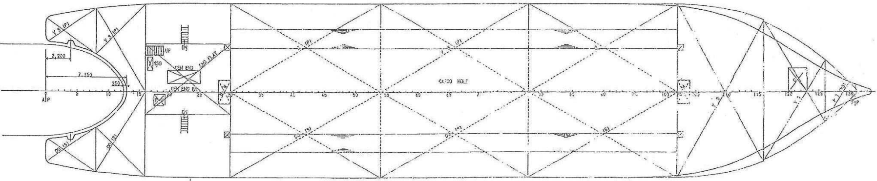
底平面 BOTTOM PLAN
