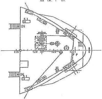
F'CLE DECK 首楼甲板
