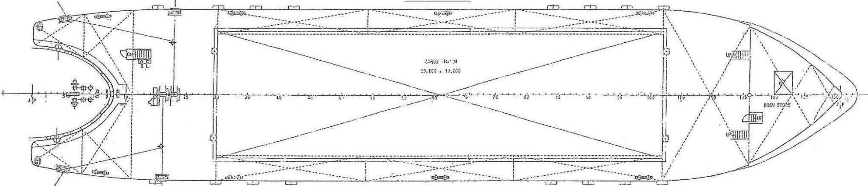
底平面 BOTTOM PLAN
